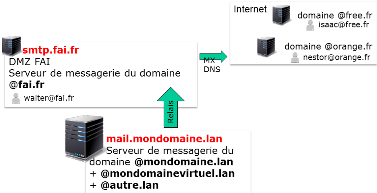
Figure 63. Système de messagerie avec relais
