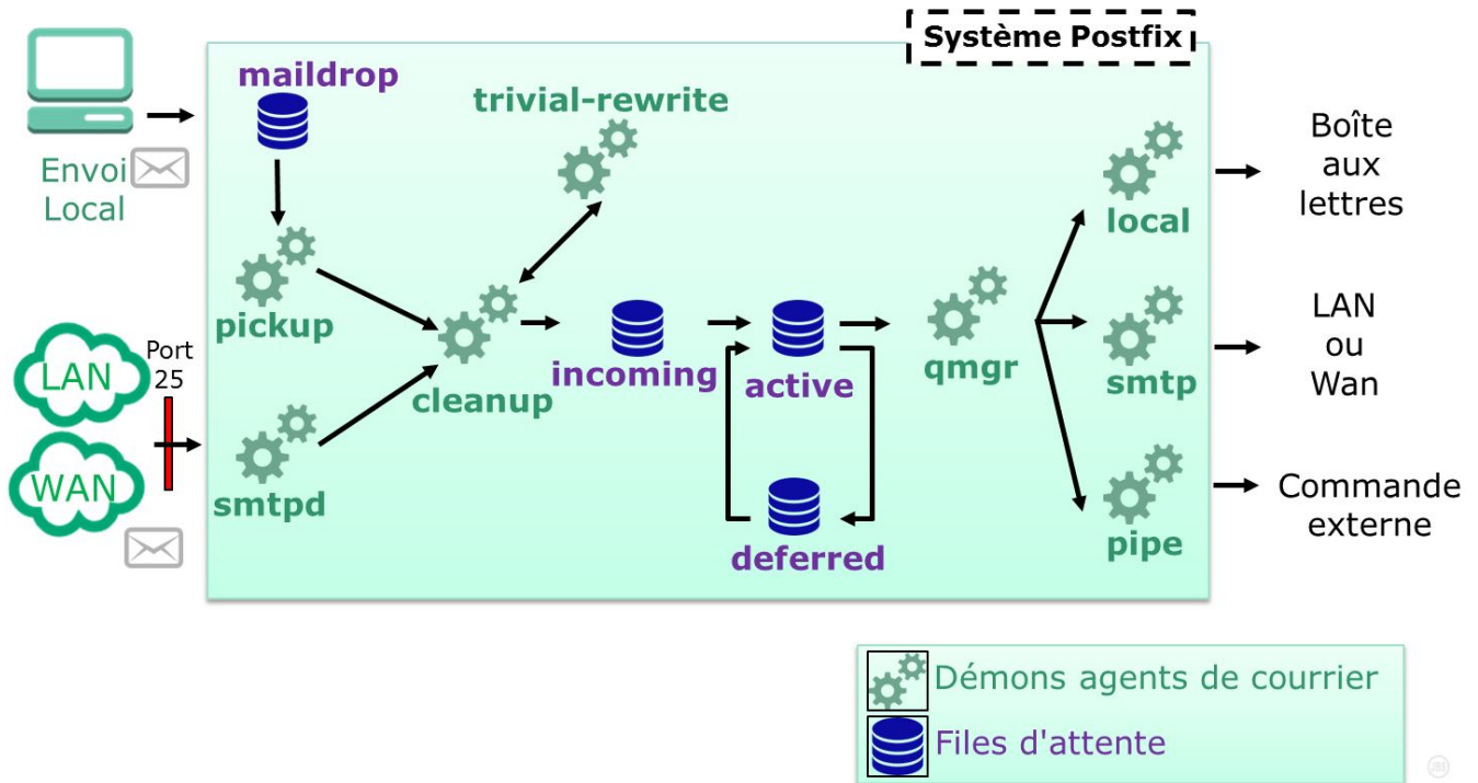
Figure 66. Synoptique global de postfix
