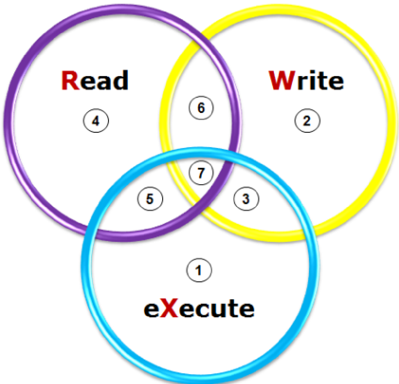
Figure 20. Méthode octale
